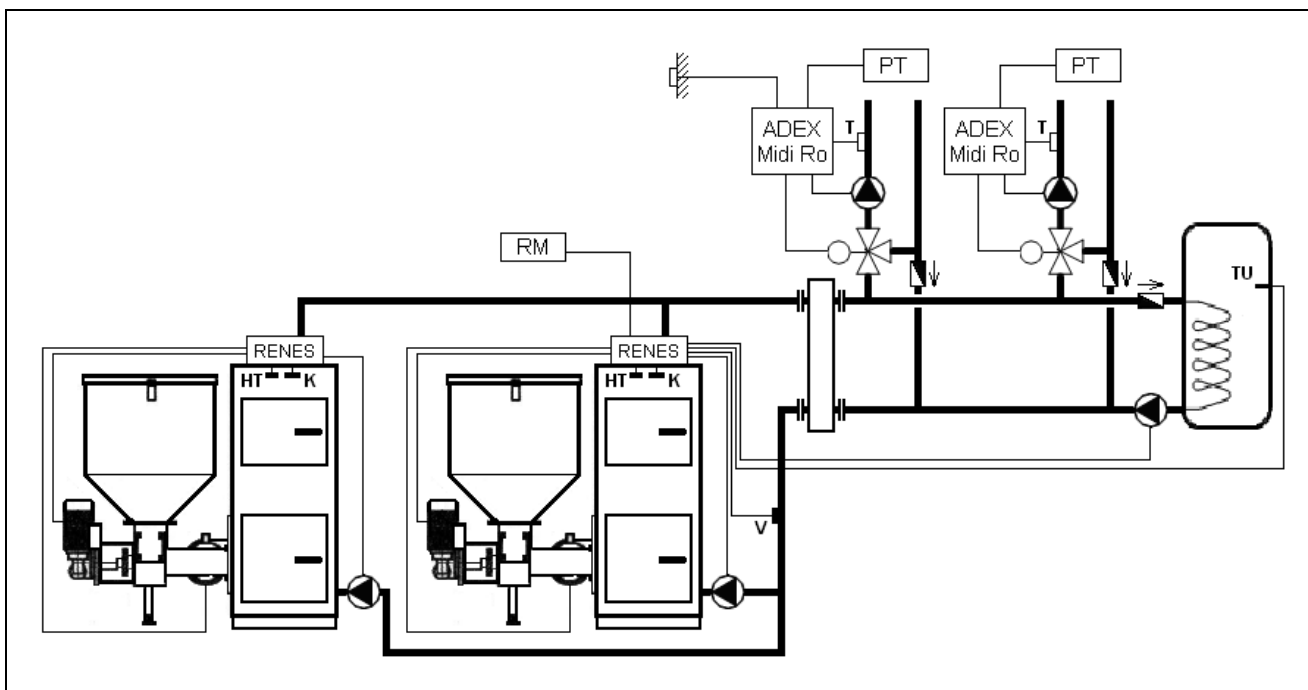
Obr. 6 Zapojení s více kotli a více topnými okruhy. U tohoto zapojení dbejte na správné dimenzování anuloidu a čerpadel. Kotle provozujte v režimu MAN nebo PROG . Má-li být zajištěn ohřev TUV, musí být v provozu kotel s radiovým modulem . Pokud přesto chcete tento kotel odstavit, přepněte jeho regulátor do režimu VYP a nechejte jej pod napětím. Měří totiž pro ostatní regulátory teplotu na čidle V .
