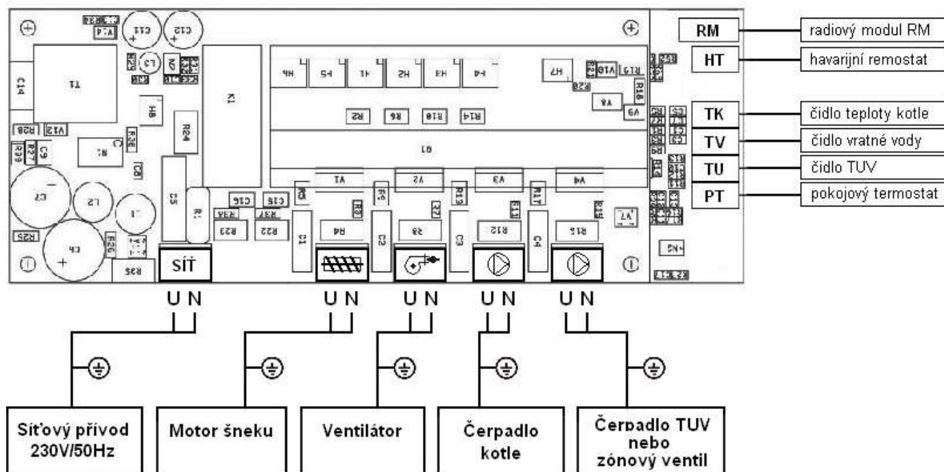
Obr. 2 Elektrické zapojení regulátoru
