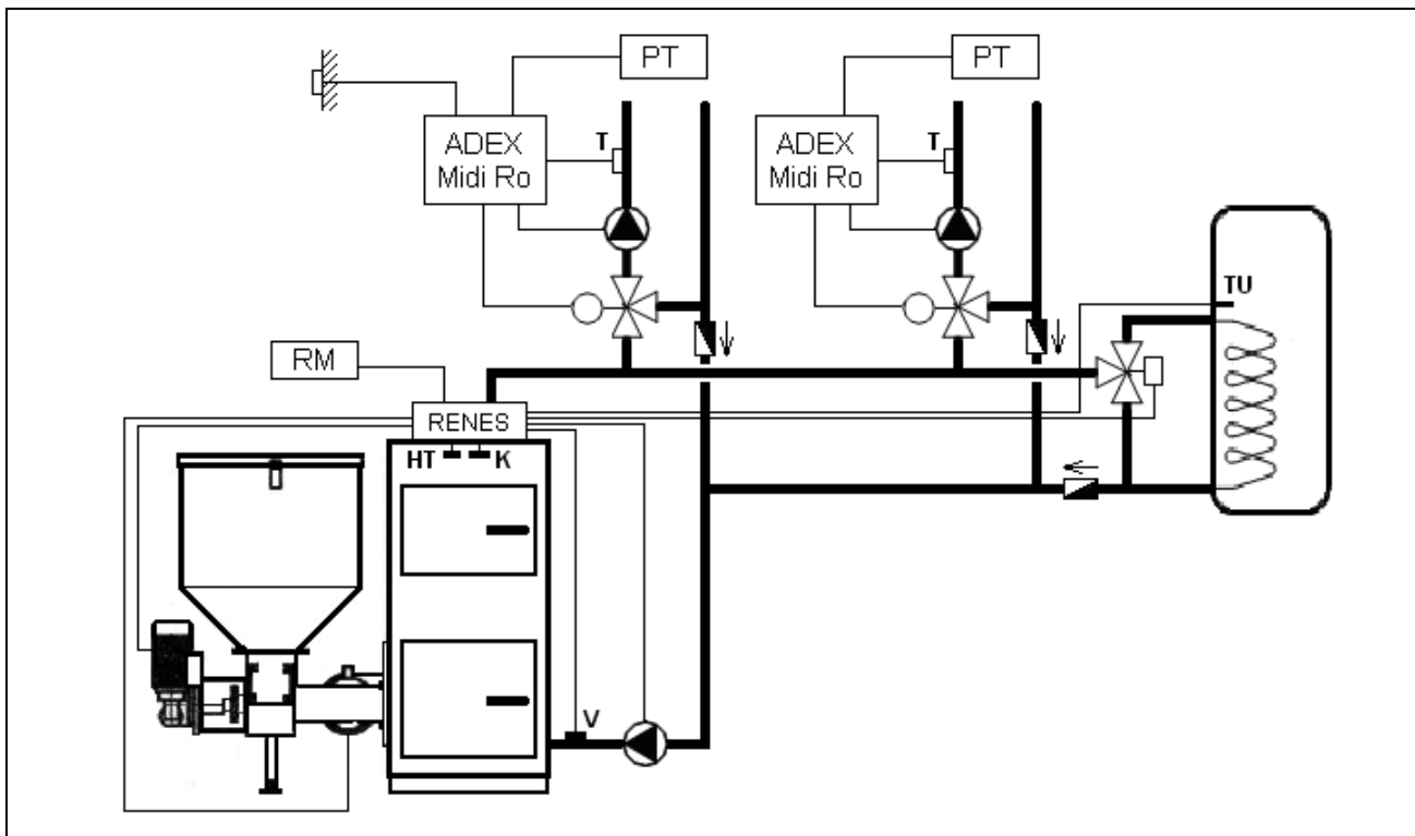
Obr. 5 Zapojení s jedním kotlem a více topnými okruhy. Provozní teploty kotle jsou regulovány automaticky podle potřeby bojleru a topných okruhů. Ohřev bojleru je řízen pomocí přepínacího ventilu.
