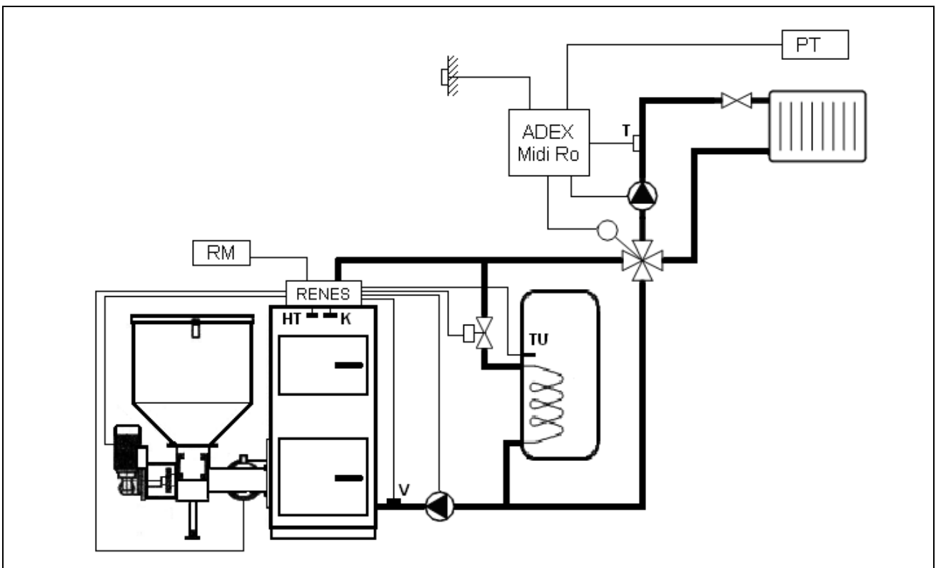
Obr. 4 Zapojení i funkce jako na obr. 3 s tím rozdílem, že je ohřev TUV regulován pomocí zónového ventilu. Zde je třeba dbát na správné dimenzování ventilů a potrubí k bojleru, aby byl přes bojler zajištěn dostatečný průtok topné vody.
